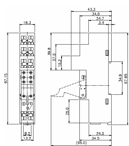
Federzugklemmen logische Trennung (C)
