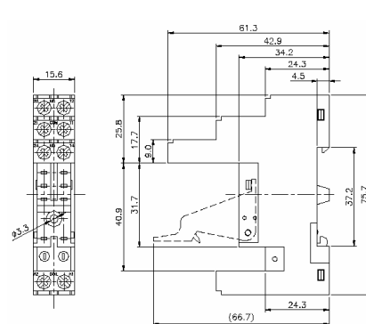
Schraubklemmen logische Trennung (T)
