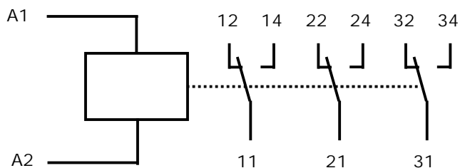
Schaltbild
